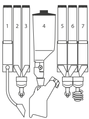
CAFÉ EN GRANO (configuración válida para versión con grupo espresso tradicional + versión con grupo de cámara variable)
