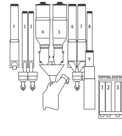
CAFFÈ IN GRANI v2 TRAMOGGE (configurazione valida per versione con gruppoespresso tradizionale + versione con gruppo caffè a camera variabile)
